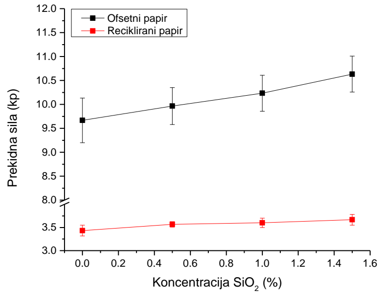
Slika 15: Vlačna čvrstoća papira tiskanih UV luminiscentnim premazima
