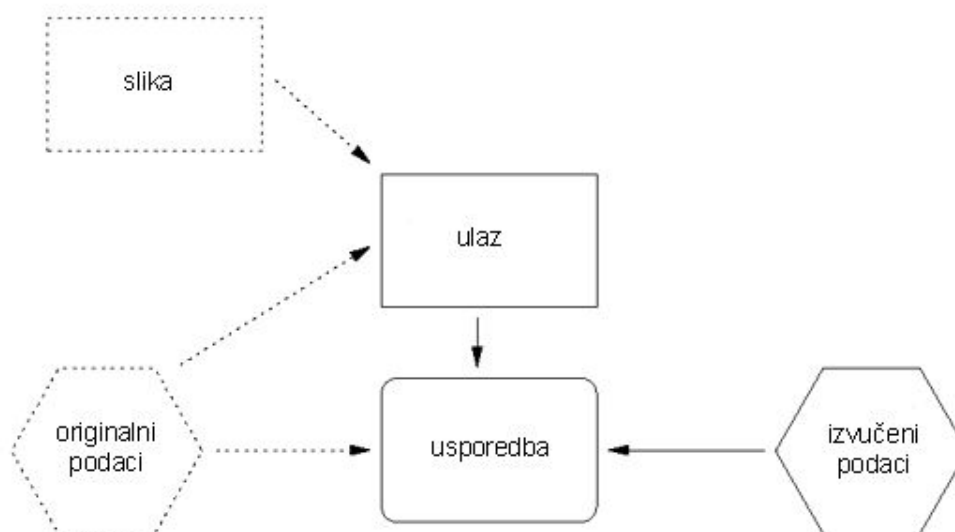
Slika 7. Shematski prikaz detekcije digitalnog vodenog žiga
