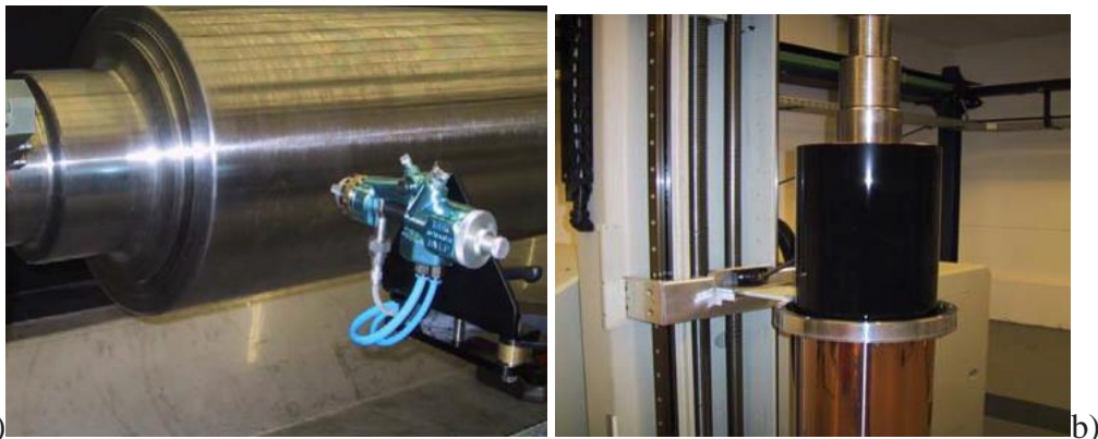
Slika 4.41 a) Oslojavanje raspršivanjem maske po površini cilindra, b) Oslojavanje uranjanjem uranjanjem cilindra radi formiranja maske[13]
