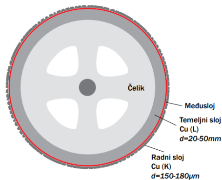
Slika 4.38 Presjek tiskovne forme za bakrotisak[13]
