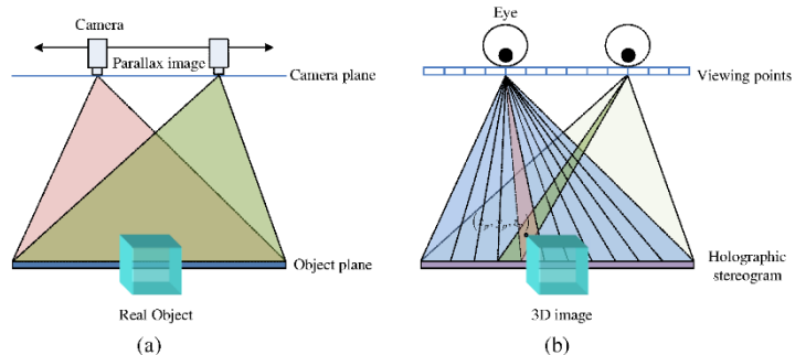
Slika 18 - holografski stereogram
