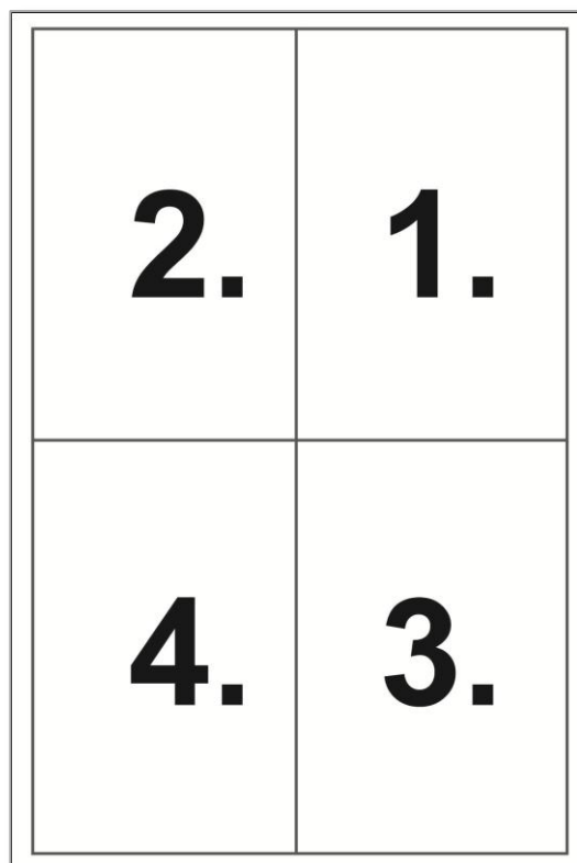
Slika 27:Optički kvadranti
