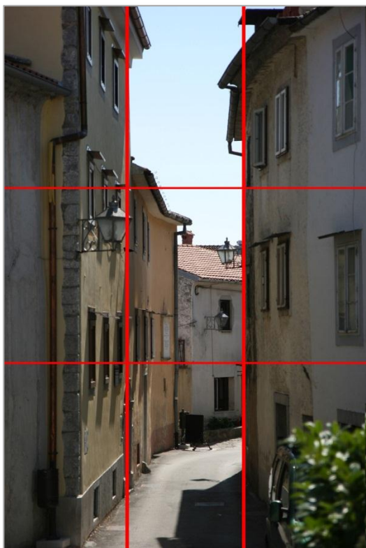
Slika 26:Pravilo tećina
