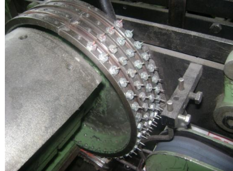
Slika 9. Perforator na ventil stroju
