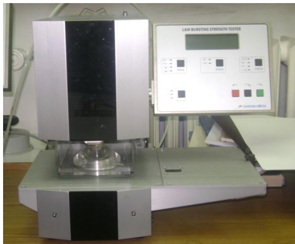
Slika 29. Uređaj Mullen
