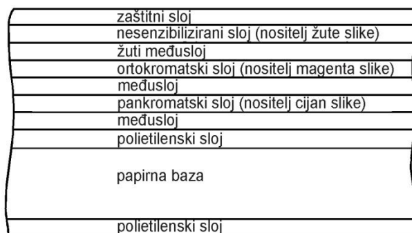
Slika 13: Prikaz slojeva fotografskog papira
