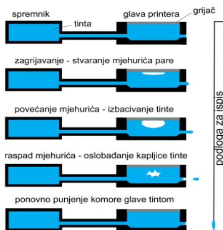
Slika 17: Princip rada ink jet pisača sa grijačem tzv. “ bubble jet ”
