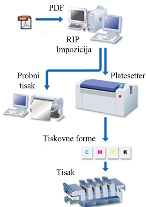
Slika 7. Radni tijek CtP sustava
