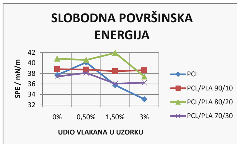
Dijagram 34 - slobodna površinska energija
