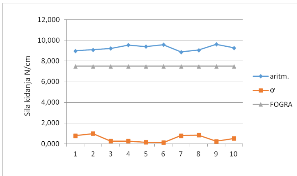
Grafikon 4. Aritmetičke sredine sile kidanja za 10 knjiga od papira Garda gloss 115 g/m 2
