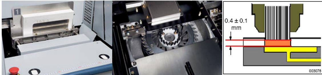
Slika 15: Prikaz uređaja za transport knjižnog blok, uređaja za piljenje i hrapavljenje hrbta sa četkama i usisavačem, dizna za nanošenje ljepila na hrbat
