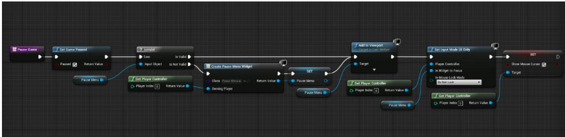
Slika 68 Funkcija PauseGame
