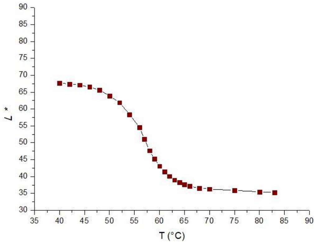
Slika 17 – L^*/T graf za Mg60 na PP
