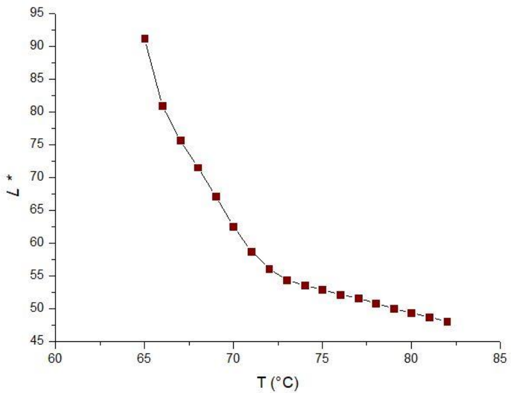
Slika 39 - L^*/T graf za THERMOSIL RED na FASSON
