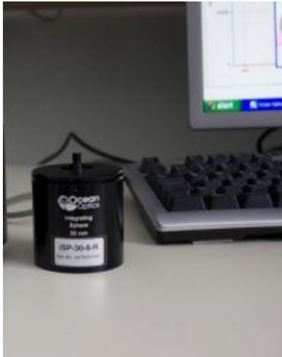
Slika 13 – Integracijska sfera OcenOptics ISP-30-6-R-GT
