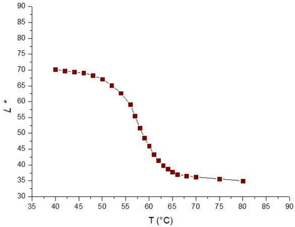
Slika 23 - L^*/T graf za Mg60 na V
