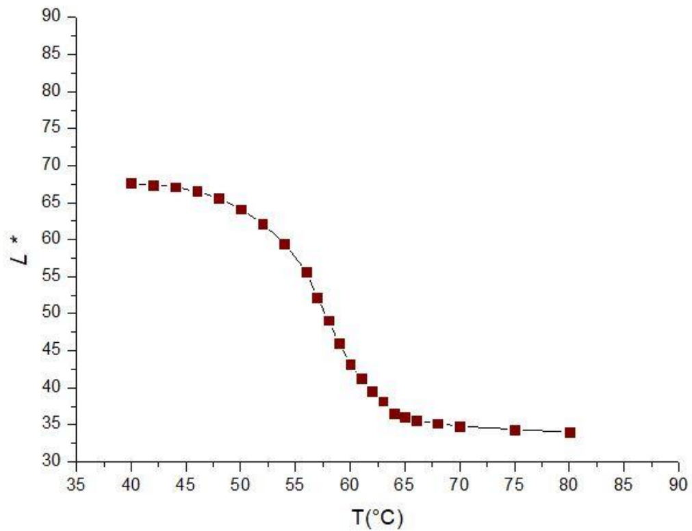
Slika 20 - L^*/T graf za Mg60 na Ni
