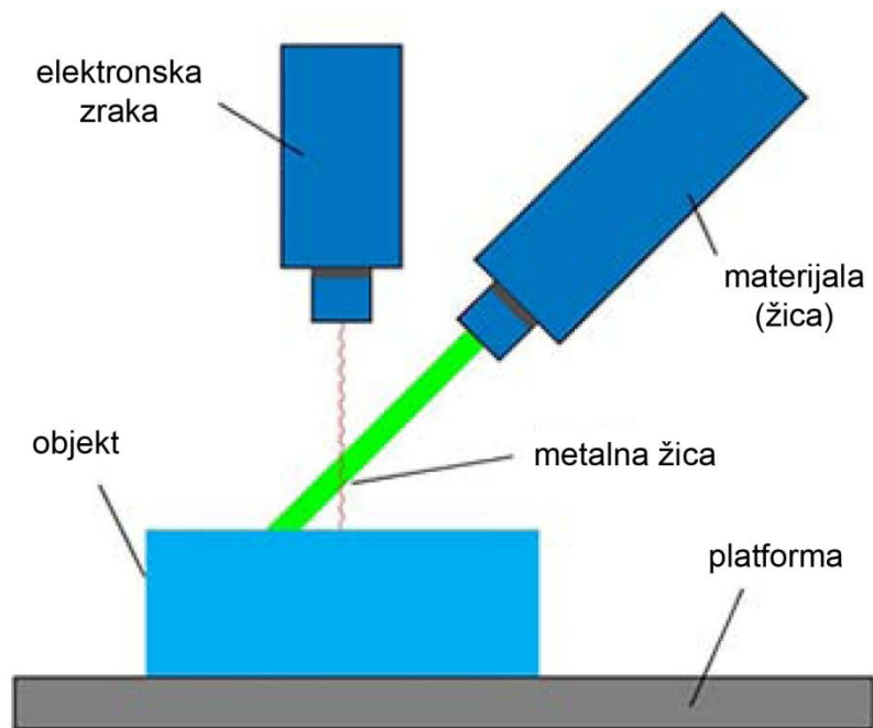
Slika 34. Prikaz DED procesa
