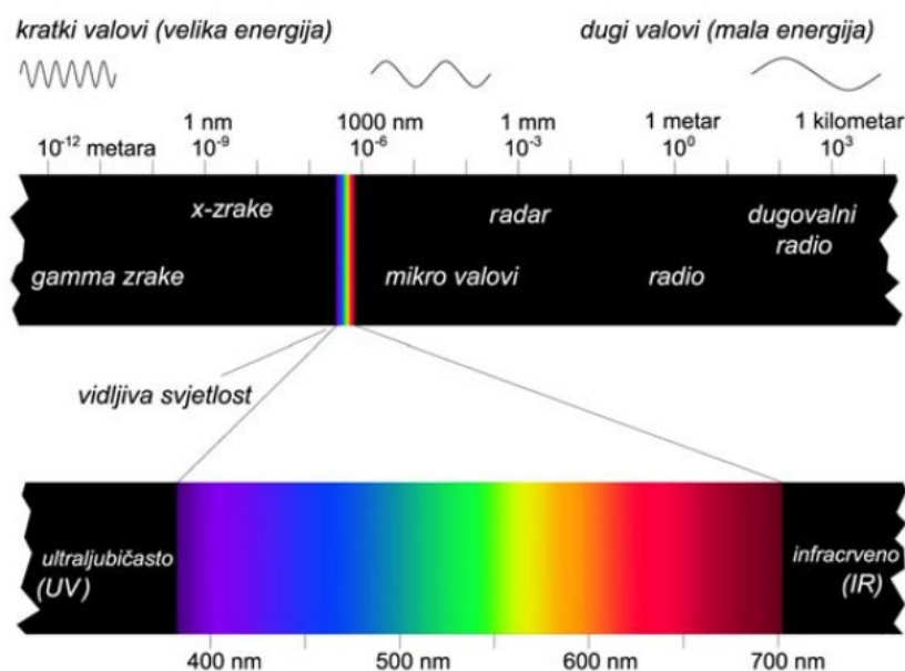
Slika 2.1. Spektar elektromagnetskih valova i vidljivog dijela spektra [6].
