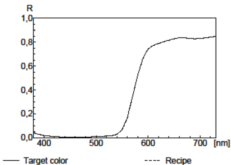
Graf 3.24. Spektralna krivulja spot narančaste 021.
