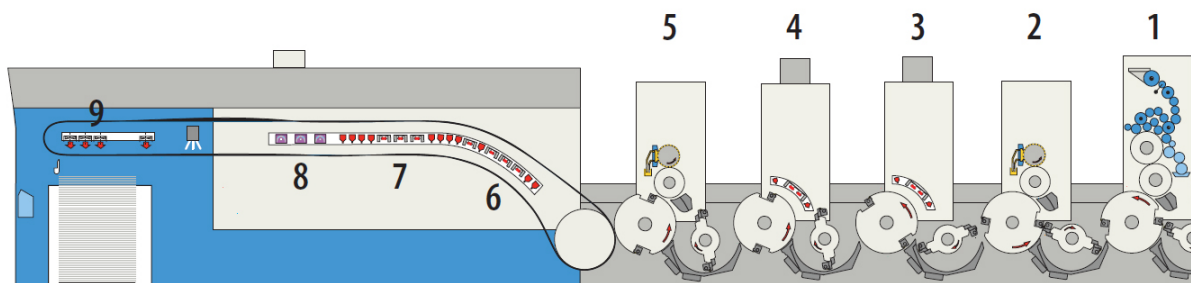
Slika 2.12. Shematski prikaz konstrukcije tiskarskog stroja prilagođenog nanosu primer laka 1) posljednja tiskovna jedinica; 2) vododisperzivna primer lak jedinica s aniloksnim valjkom; 3,4) dvije jedinice namijenjene sušenju vododisperzivnog laka IR zračenjem i vrućim zrakom; 5) lak jedinica za nanošenje UV laka; 6,7) produljeni izlagači aparata tiskarskog stroja opremljeni IR sušenjem i sušenjem vrućim zrakom; 8) jedinica za UV-A/B/C zračenje; 9) sustav za otklanjanje preostalog ozona i pudera [24]
