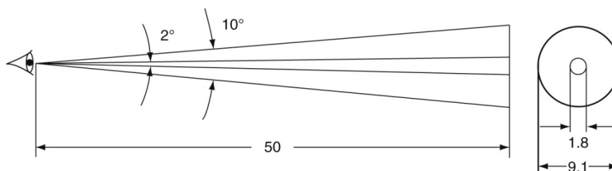
Slika 2.37. Prikaz veličine uzorka i udaljenost kod CIE 1931 i CIE 1964 standardnog promatrača ( 2^\circ i 10^\circ )
