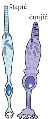
Slika 2.10. Prikaz fotoreceptora štapića i čunjića
