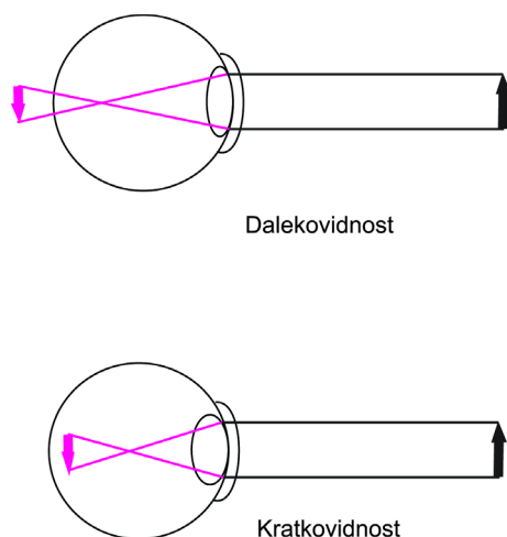
Slika 2.14. Prikaz dalekovidnosti i kratkovidnosti
