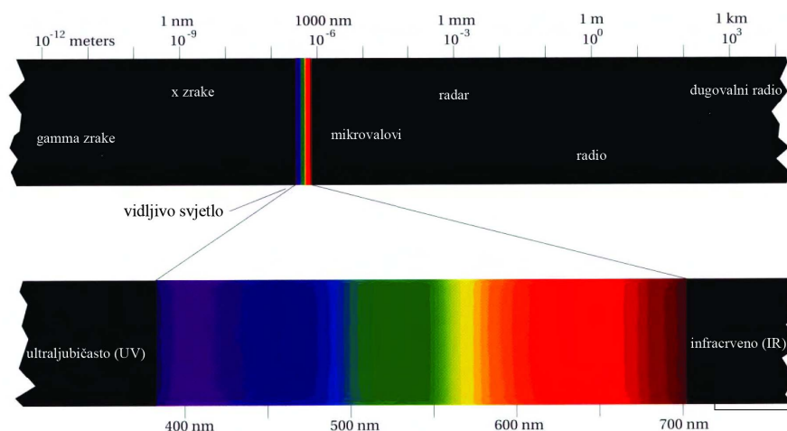
Slika 2.21. Prikaz spektra boja
