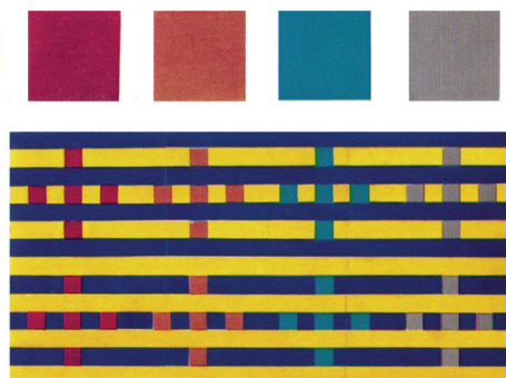
Slika 2.56. Prikaz Gindyevog efekta
