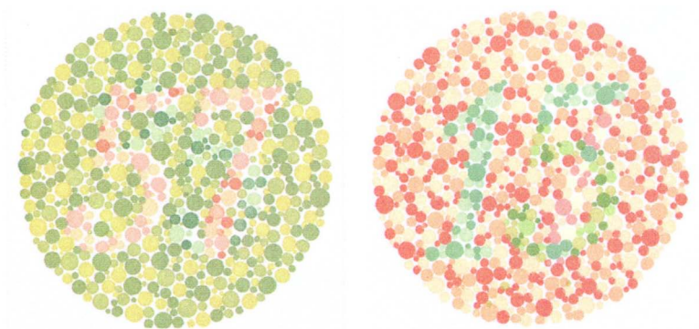
Slika 2.20. Ishihara test za slijepilo na boje (Dvije ploče koje se koriste za test slijepila na boje. Na lijevoj ploči osobe koje ne raspoznaju crveno-zeleno obojenje vide broj 5; dok jedni vide broj 7; a ostali ne vide ništa. Isto tako kod desne ploče osobe s normalnim vidom vide broj 15, dok osobe koje ne raspoznaju crveno-zeleno obojenje ne vide nijedan broj)
