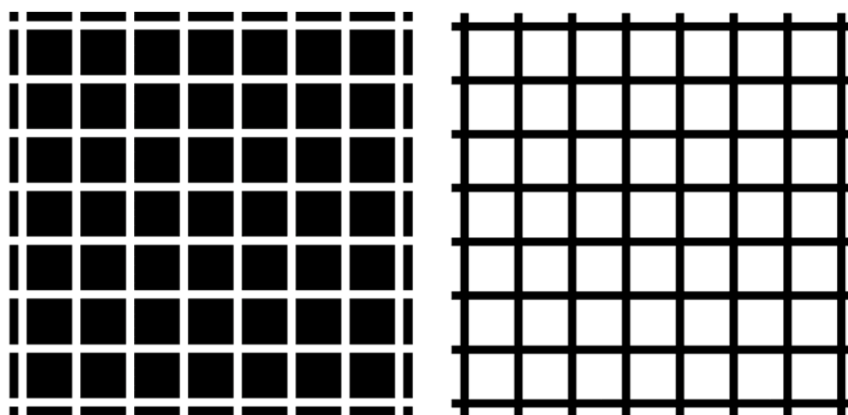
Slika 2.44. Hermannov efekt
