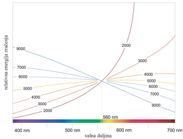
Slika 2.36. Spektralna emisija različitih temperatura crnog tijela u dijelu spektra od 400 do 700 nm tako a svi imaju istu vrijednost kod 560 nm
