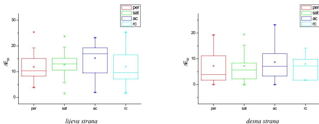
Slika 4.11. Intenzitet efekata u ovisnosti o standardnim metodama renderiranja za primarni stimulus plave boje i sekundarni stimulus čijan i magenta boje na lijevoj strani (laboratorijski uvjeti, metoda simultano binokularno usuglašavanje)
