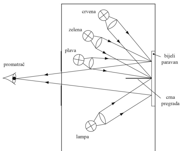
Slika 2.24. Vizualni tristimulusni eksperiment
