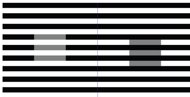
Slika 2.53. Whiteov efekt
