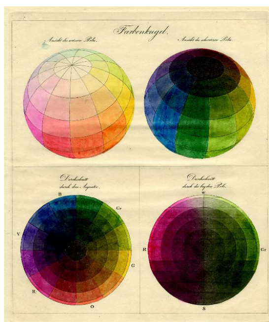
Slika 2.31. Rungeov sustav boja
