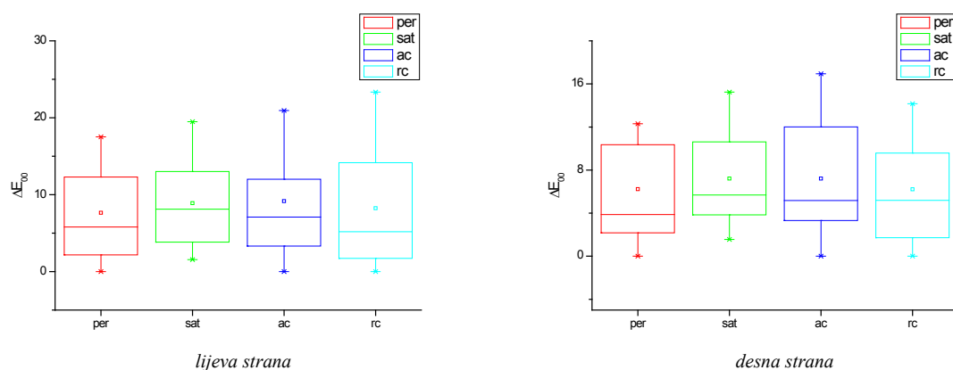
Slika 4.47. Intenzitet efekata u ovisnosti o standardnim metodama renderiranja za primarni stimulus plave boje i sekundarni stimulus cijan i magenta boje na lijevoj i desnoj strani (realni uvjeti, metoda simultano binokularno usuglašavanje)
