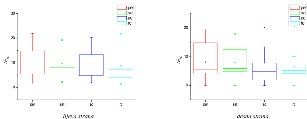
Slika 4.48. Intenzitet efekata u ovisnosti o standardnim metodama renderiranja za primarni stimulus crvene boje i sekundarni stimulus žute i magenta boje na lijevoj i desnoj strani (realni uvjeti, metoda simultano binokularno usuglašavanje)
