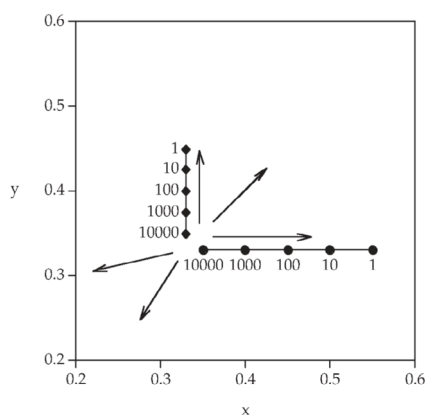
Slika 2.48. Prikaz rezultata Huntovog vizualnog eksperimenta gdje točke odgovaraju boji za različite nivoe adaptacije. Rezultat pokazuje da je potrebna osjetljivost niske čistoće pobude kod 10000 \text{ cdm}^{-2} uskladi sa stimulusom visoke čistoće pobude promatran pod 1 \text{ cdm}^{-2}
