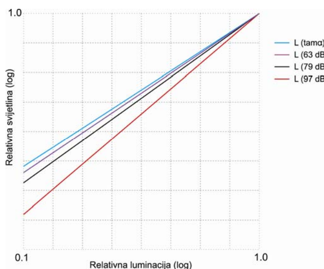
Slika 2.34. Stevensov efekt [26]
