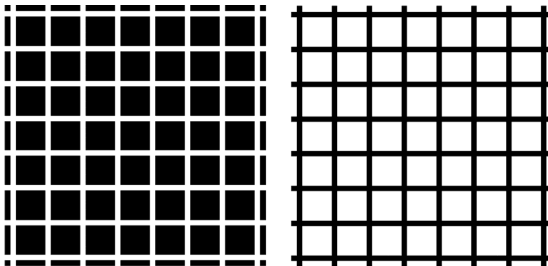
Slika 2.28. Hermannov efekt [86]
