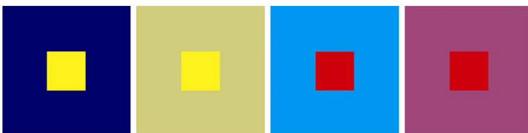
Slika 2.18. Kromatski simultani kontrast [66]
