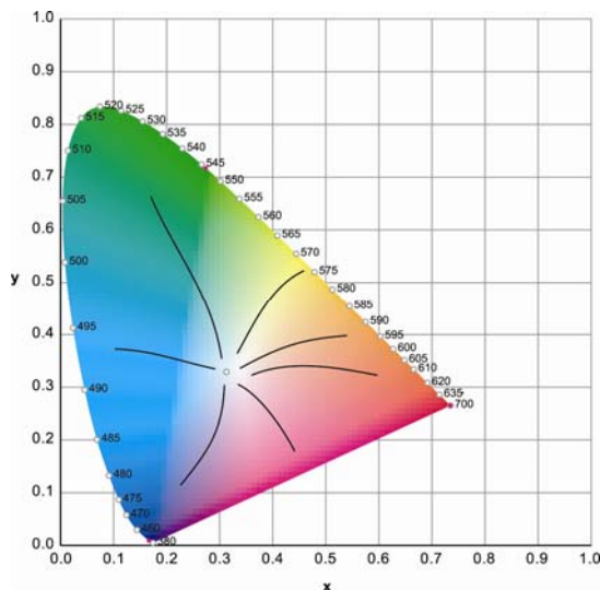
Slika 2.32. Abneyev efekt unutar CIE dijagrama kromatičnosti [66]
