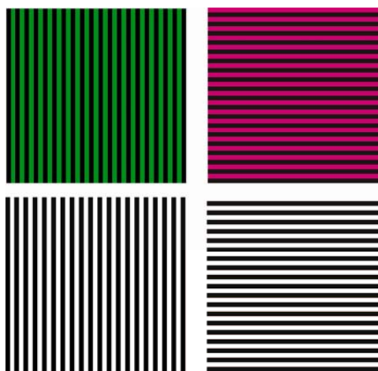
Slika 2.27. Prikaz McCollough efekta [26]
