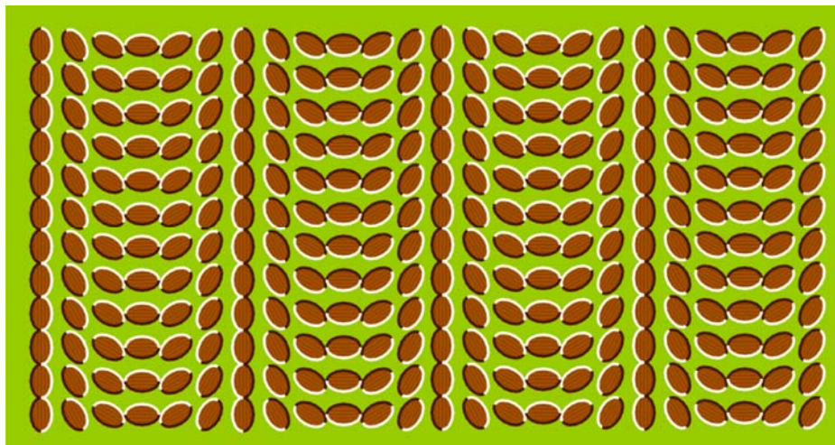
Slika 2.29. „Donguri“ uzorak [107]
