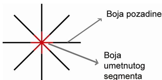
Slika 2.35. Ehrenstein model
