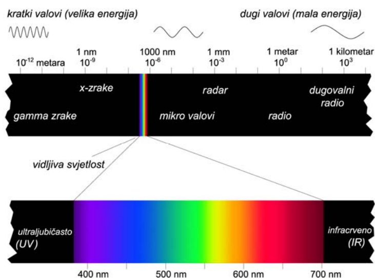
Slika 2.4. Spektar elektromagnetskih valova i vidljivog dijela spektra [29]
