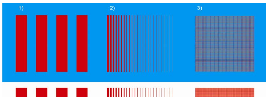
Slika 2.23. Proširivanje boje [66]
