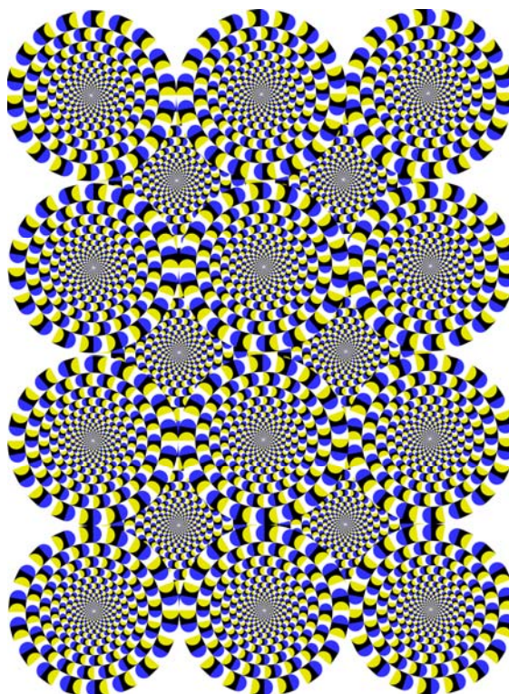
Slika 2.30. „Roto-Snakes“ efekt [107]
