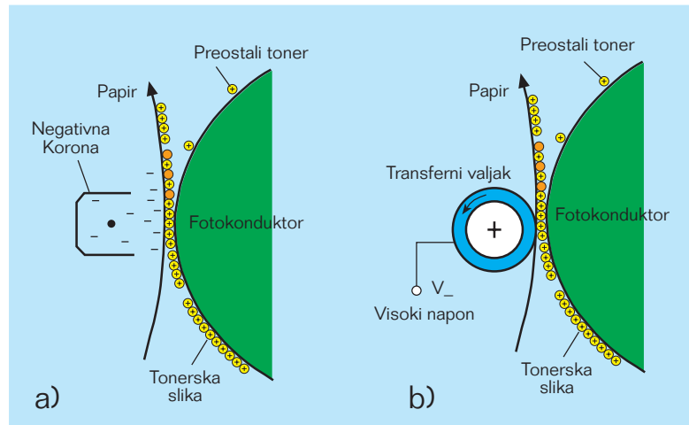
Slika 31. Konstrukcija uređaja za direktno prenošenje tonera na papir
