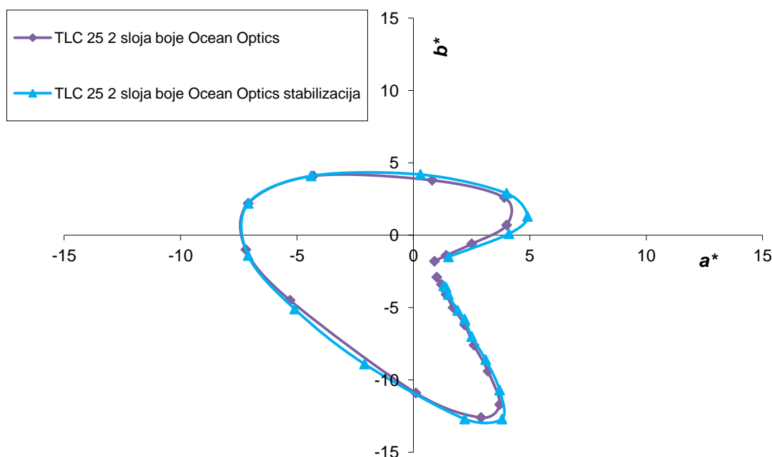
Slika 41. Usporedba kromatičnih vrijednosti TLC 25 tiskarske boje sa i bez stabilizacije temperature tijekom mjerenja, prikazane u CIELAB ( a^*b^* ) dijagramu
