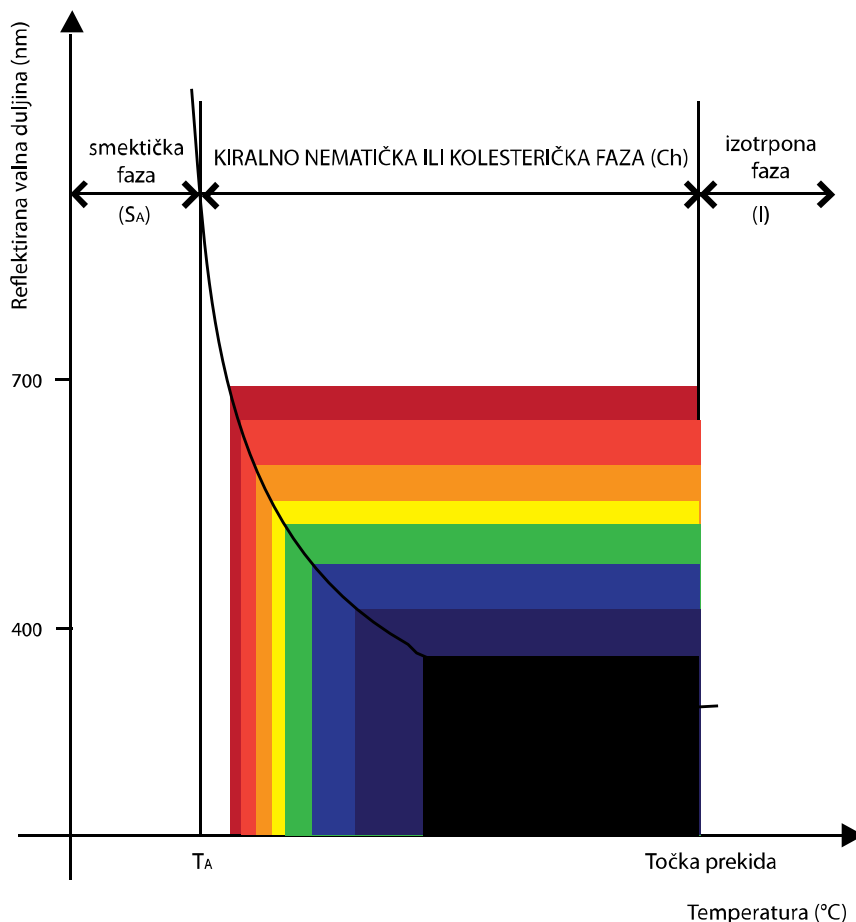
Slika 6. Karakteristične valne duljine reflektirane svjetlosti tekućih kristala u ovisnosti o temperaturi (Stasiek i Kowalewski, 2002; Stasiek et al. , 2006)
