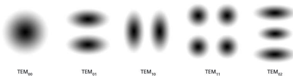
Slika 14. Primjeri Hermite- Gaussovih modova nižeg reda
