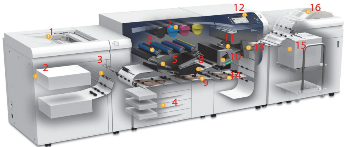
Slika 13 – dijelovi stroja [8]
