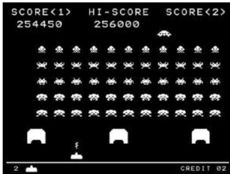
Slika 2. Space Invaders
