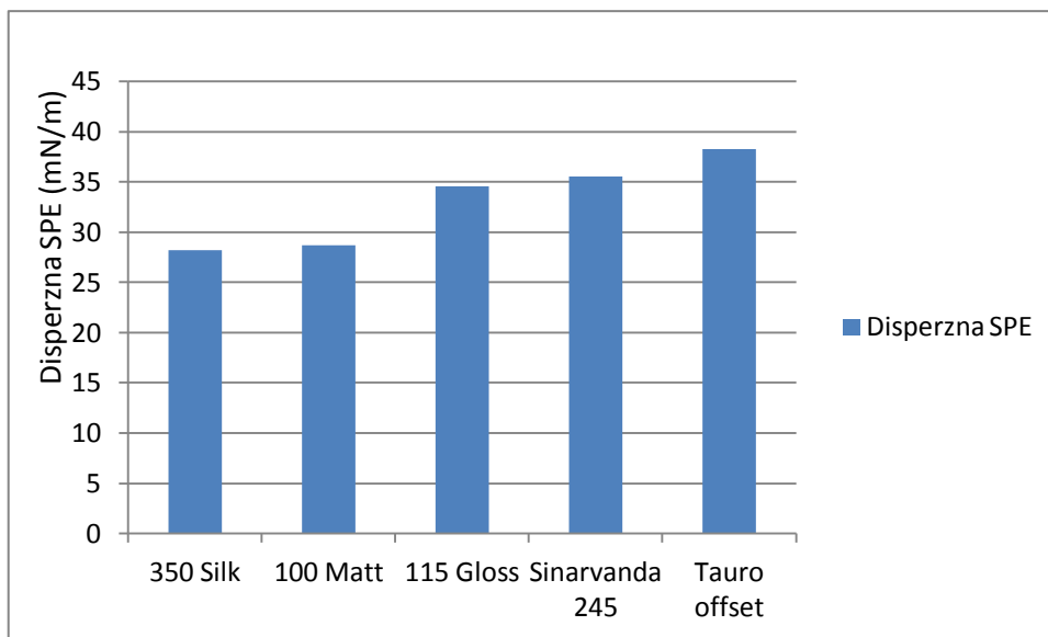
Slika 34. Dispersna komponenta SPE
