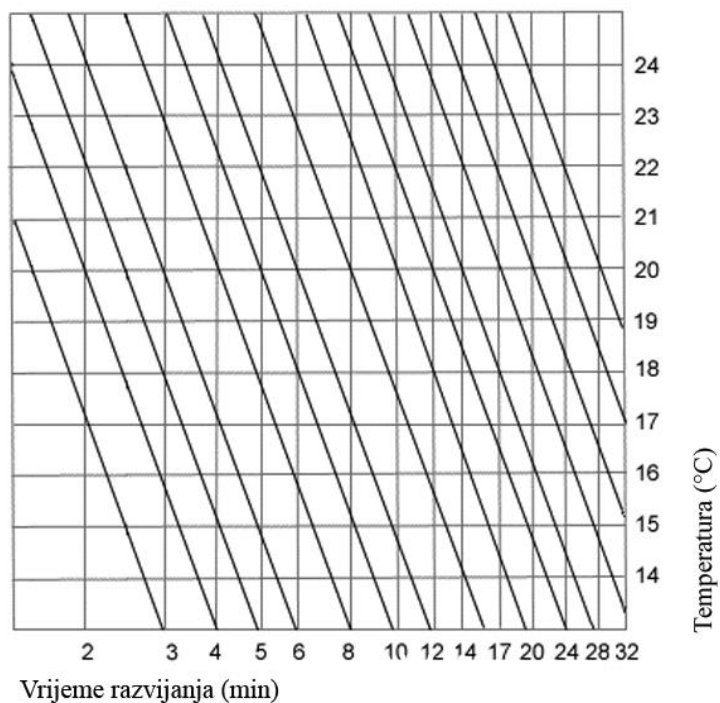
Slika 3: Ovisnost vremena razvijanja o temperaturi razvijачa
