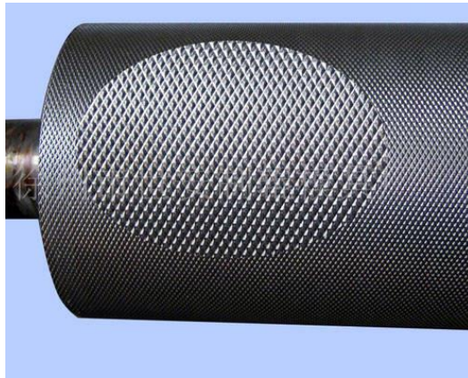
Slika 3. Aniloks cilindar
