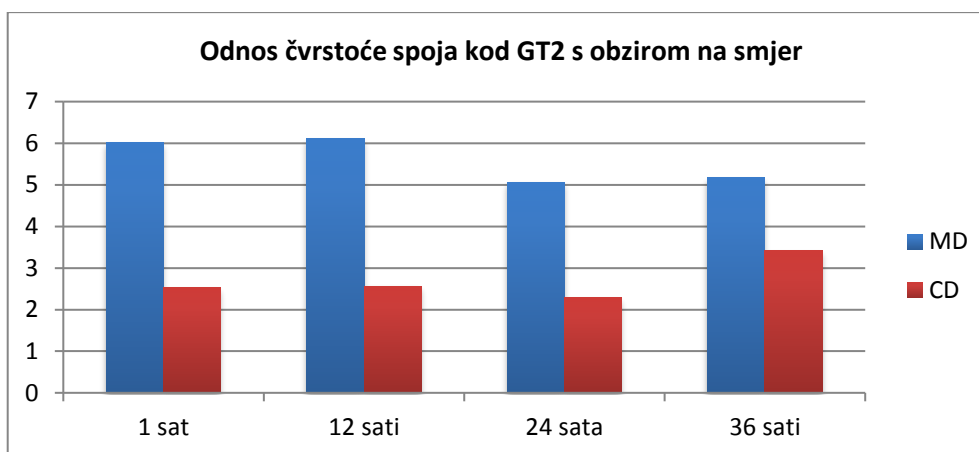
Grafikon 9.: Prikaz vrijednosti čvrstoće ispitanog spoja s obzirom na smjer tok vlakana kod kartona GT2
