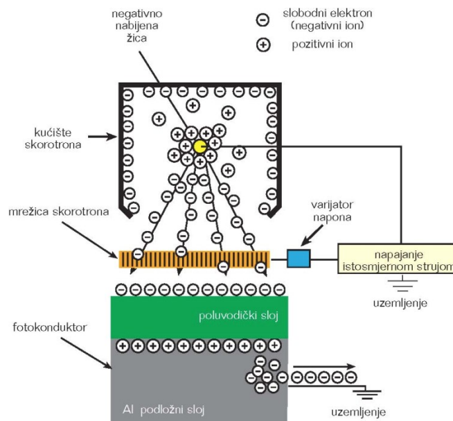
Slika 5. Princip negativskog nabijanja (Izvor: I. Majnarić, Studija indirektno elektrografije, doktorska disertacija, 2007.)
