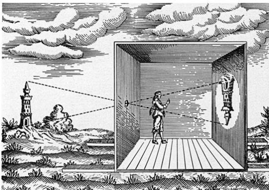
Slika 1. Camera obscura
