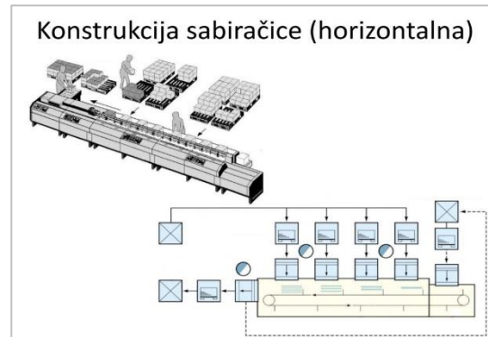
Slika 35. Vertikalna i horizontalna sabiračica
