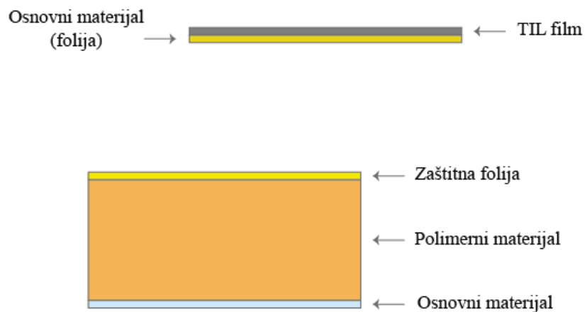
Slika 10. TIL film i tiskovna forma za TIL postupak
