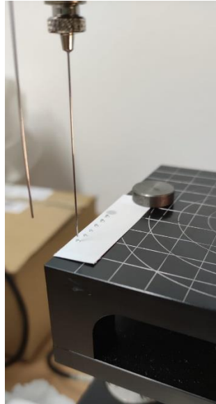
Slika 29. Prikaz postupka mjerenja kontaktnih kuteva
