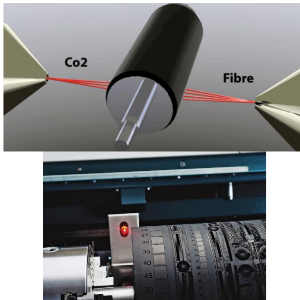
Slika 4.26 a) Lasersko graviranje ovojne tiskovne forme, b) CtP Laserska izrada tiskovne forme[13]
