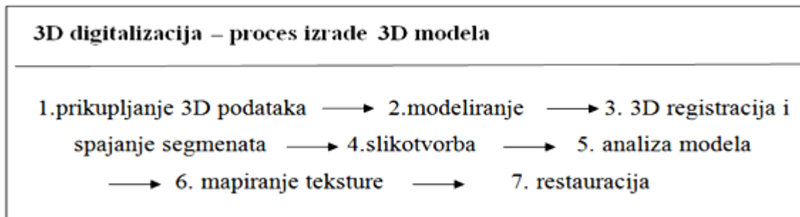
Slika 1. Postupak digitalizacije 3D modela skeniranjem
