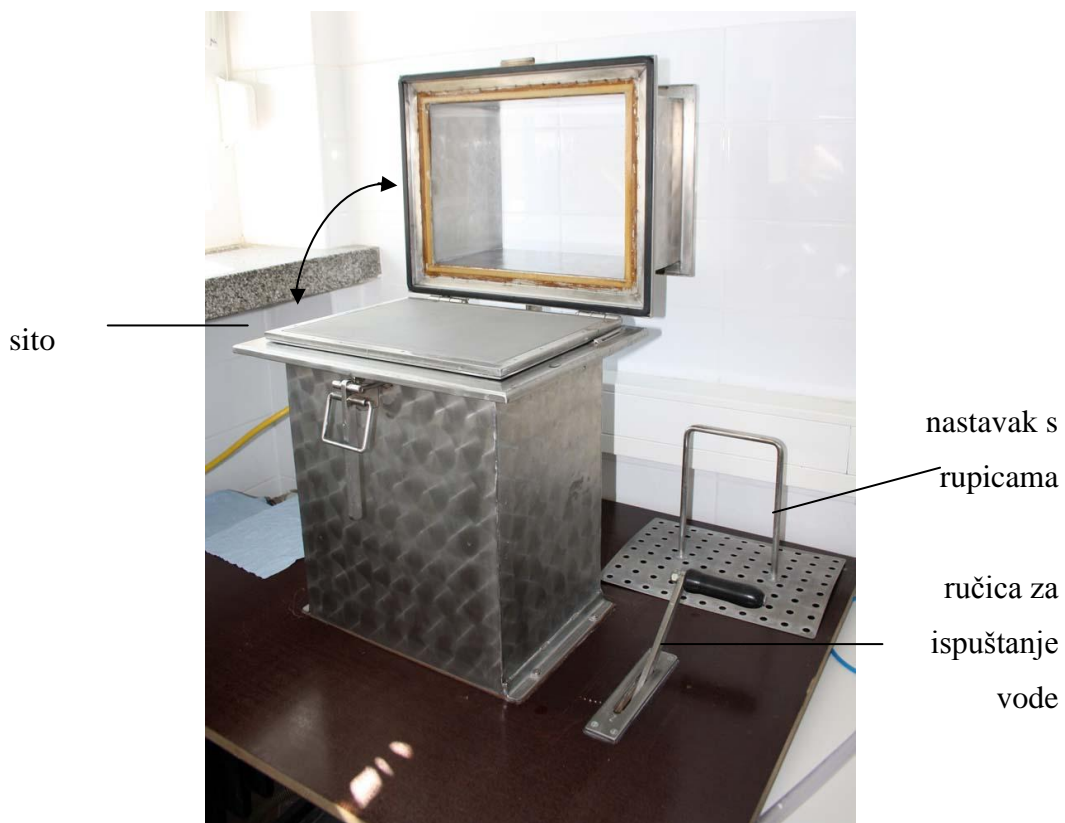
Slika 13. Uređaj za formiranje lista papira
