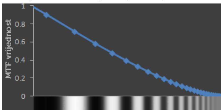
Slika 28. MTF graf za "savršeni" objektiv
