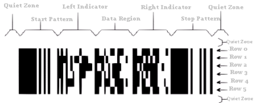
Slika 16 - struktura koda PDF417
