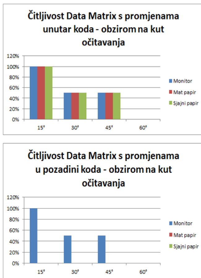
Slika 52 - grafički prikaz čitljivosti Data Matrix koda s promjenama unutar i u pozadini koda obzirom na kut očitavanja
