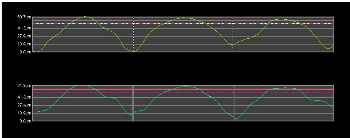
Slika 25. Presjek tiskovnih elemenata od 1% na tiskovnoj formi izrađenoj prema 10. bump up krivulji
