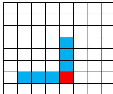
Slika 7 - Predviđanje blokova
