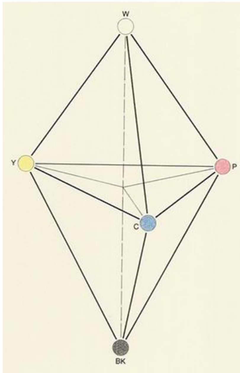
Slika 5 Mayerov tetraedar
