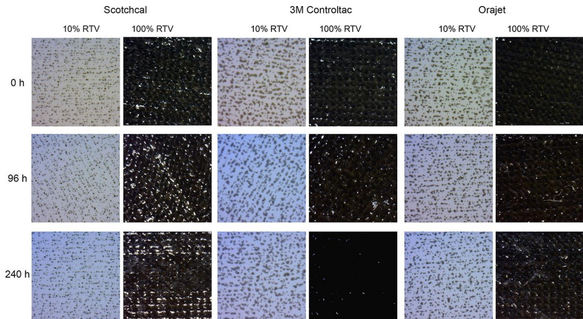
Slika 59. Mikroskopske snimke otisnutih crnih UV sušućih Inkjet uzoraka na tri Wrap folije, u periodima starenja od 0 h, 96 h i 240 h
