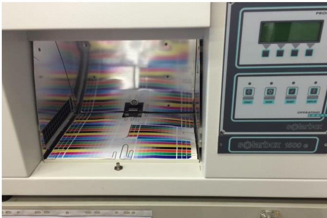
Slika 29. Solar Box komora za starenje uzoraka
