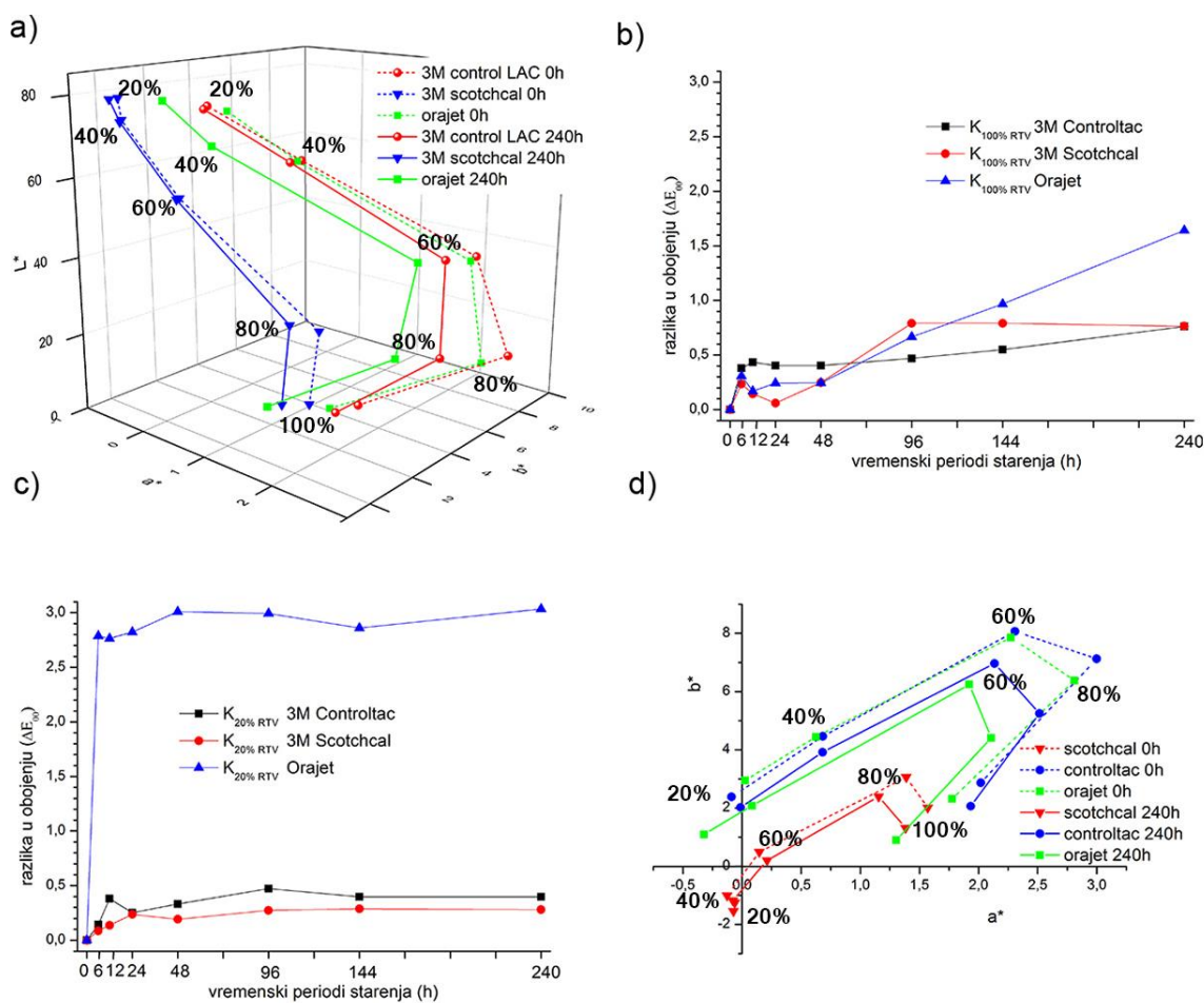
Slika 60. Promjene crne UV sušće Inkjet boje nakon 0 i 240h; a) L^*a^*b^* vrijednosti; b) \Delta E_{00} za polja od 20% RTV; c) \Delta E_{00} za polja od 100% RTV; d) promjena a^*b^* vrijednosti
