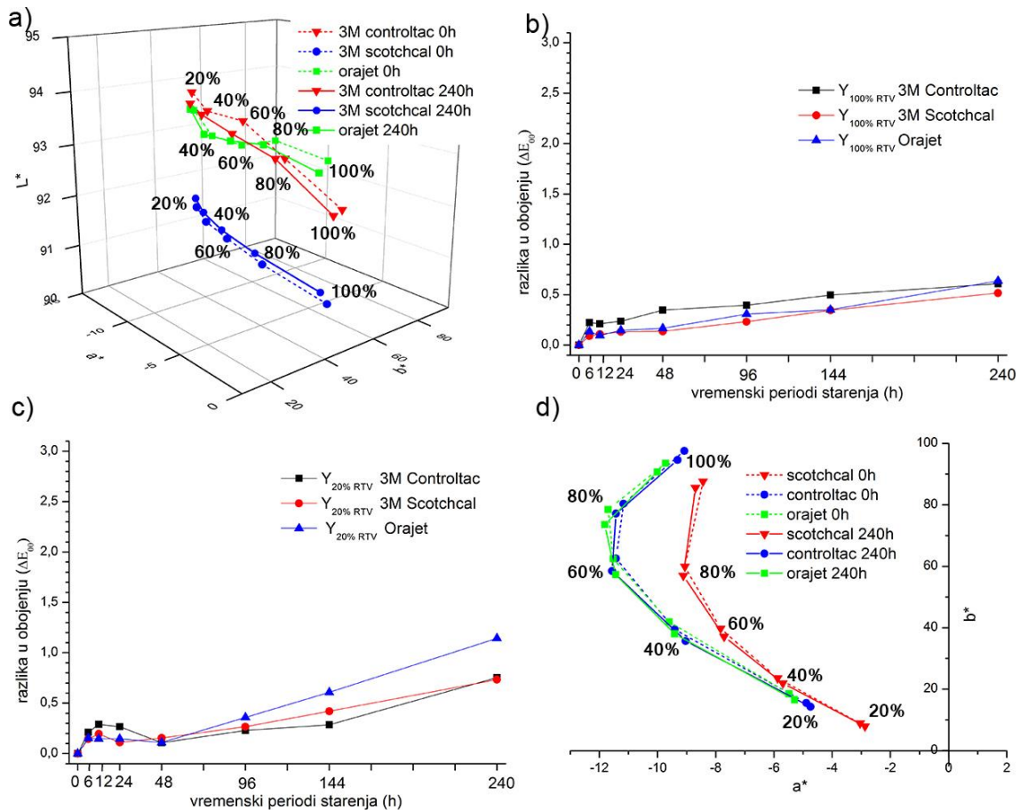
Slika 50. Promjene žute solventne Inkjet boje nakon 0 i 240h; a) L^*a^*b^* vrijednosti; b) \Delta E_{00} za polja od 20% RTV; c) \Delta E_{00} za polja od 100% RTV; d) promjena a^*b^* vrijednosti
