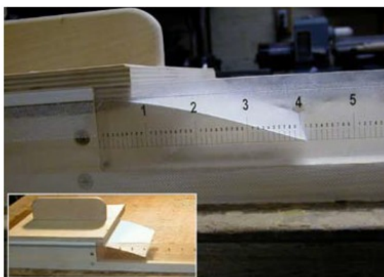
Slika 6. Uređaj Pete Jermanna za mjerenja Drape faktor
