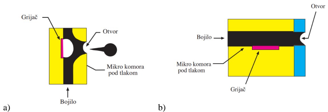
Slika 4. Konstrukcija termalne glave za inkjet: a) princip vršnog okidanja, b) princip bočnog okidanja (Izvor: I. Majnarić, Osnove digitalnog tiska, 2015.)
