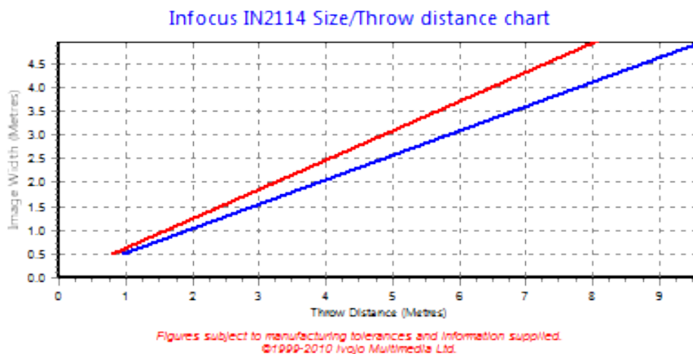
Graf 1. Povećanjem udaljenosti projektora i zida, slika se rasteže i smanjuje se rezolucija
