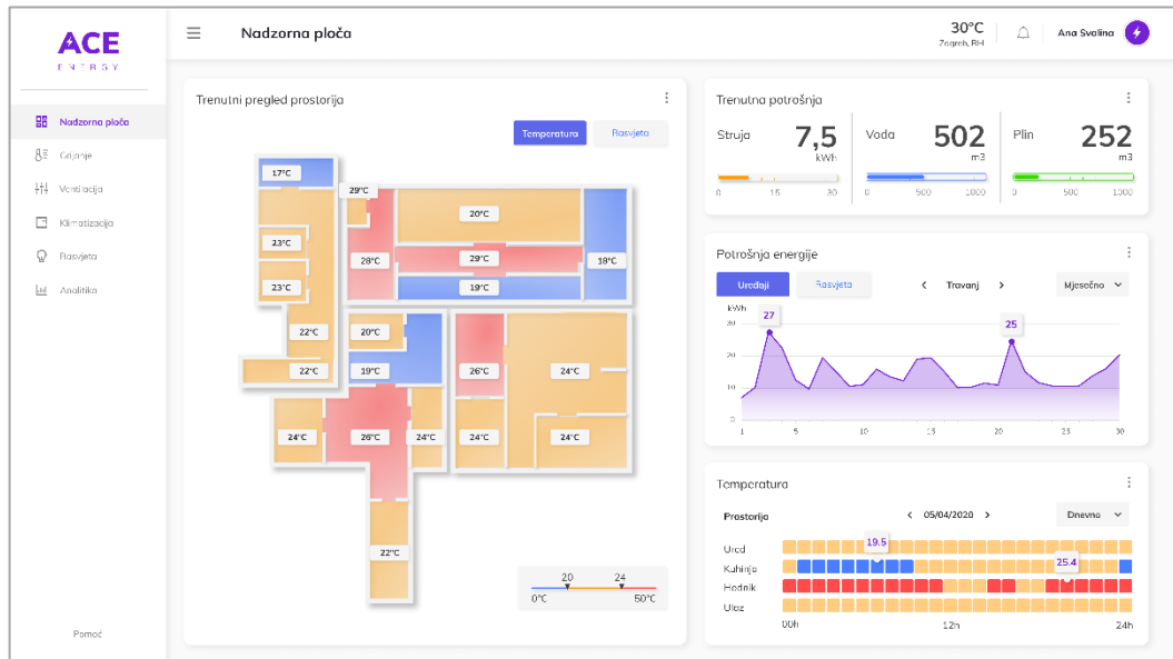
Slika 65: Krajnji prijedlog nadzorne ploče za BMS, prikaz temperatura
