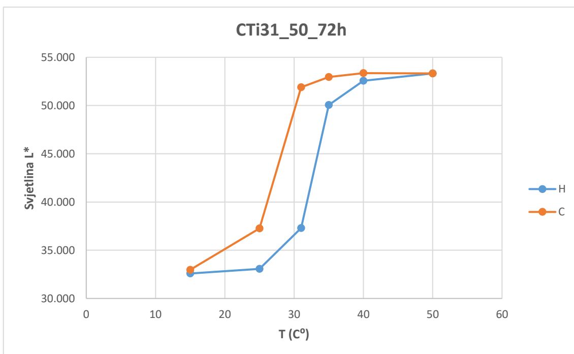
Slika 67. Ovisnost svjetline ( L^* ) o temperaturi (T) kod uzorka otiska boje CTI31 izloženog temperaturi od 50^{\circ}\text{C} na 72 sati (H- proces zagrijavanja, C- proces hlađenja)
