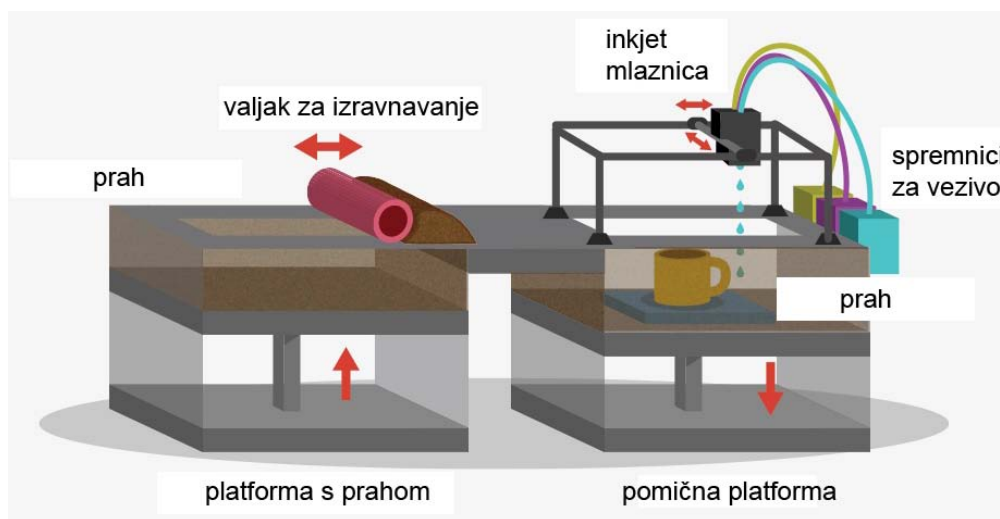
Slika 26. Prikaz Binder Jetting procesa
