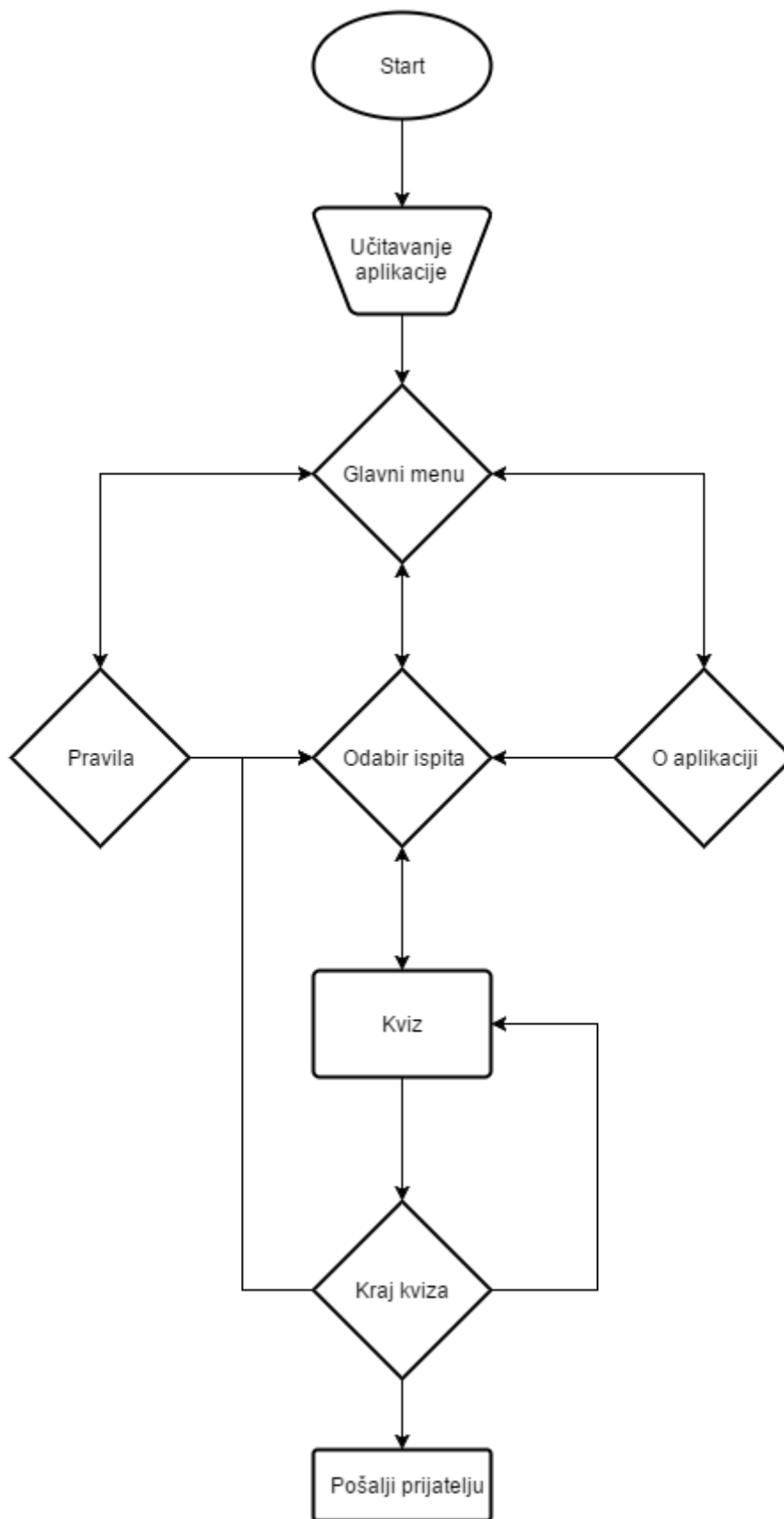
Slika 8: Dijagram toka aplikacije
