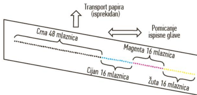
Slika 5 Segment generiranja jednog reda ispisne glave (Izvor: Majnarić, I. (2015) Osnove digitalnog tiska. Zagreb, Grafički fakultet Sveučilišta u Zagrebu.)
