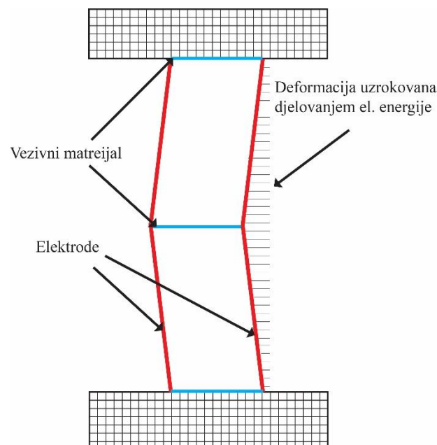
Slika 10 Prikaz deformacije uzrokovane djelovanjem električne energije
