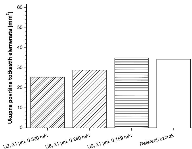
Slika 77 Grafički prikaz površina točkastih elemenata promjera 0,75 mm različitim brzinama nanosa laka
