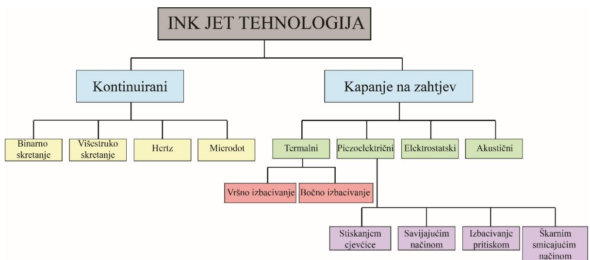
Slika 7 Prikaz podjele Inkjet tehnologija
