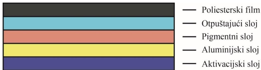
Slika 40 Presjek folije korištene u eksperimentu
