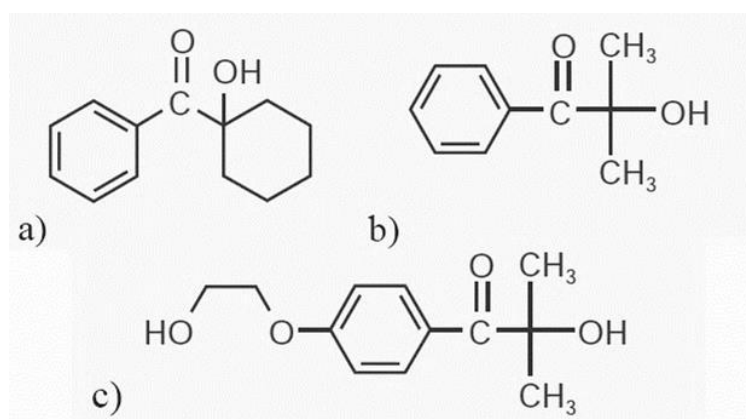
Slika 19 Kemijska struktura najčešćih fotoinicijatora; a) 1-hidroksi-cikloheksil-fenil-ke-ton; b) 2-hidroksi-2-metil-1-fenil-1-propanon); c) 2-hidroksi-1-[4-(2-hidroksi etoksi)fenil]-2-metil-1-propanon (Izvor: Katalog fotoinicijatora Ciba Speciality Chemicals)
