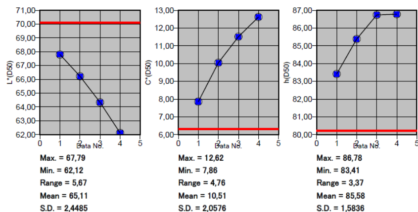
Slika 218 Prikaz svjetline, kromatičnosti i tona ispitnih uzoraka 1,0 mm - 1,8 mm
