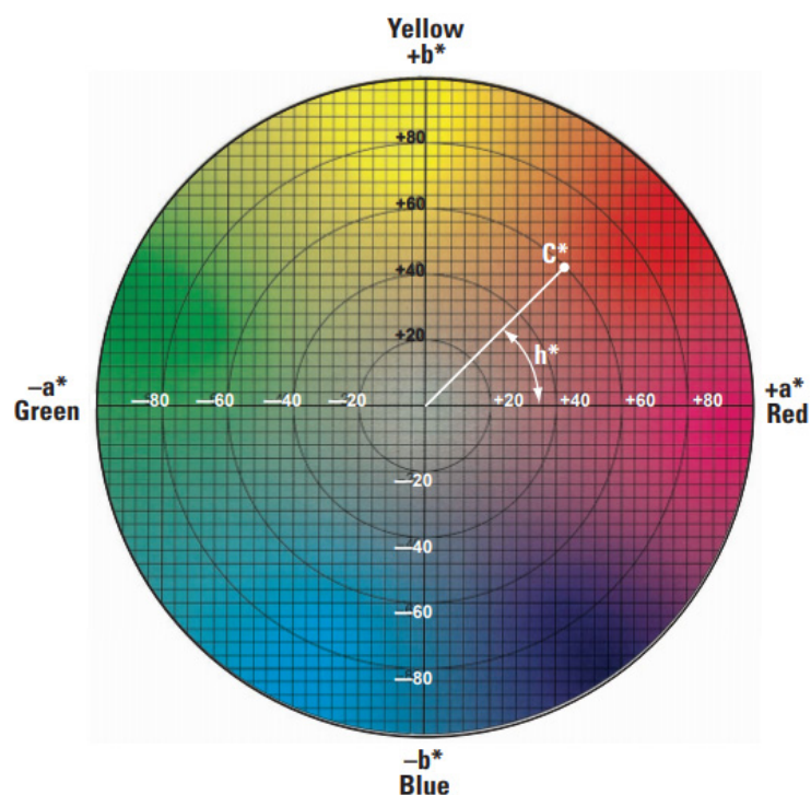
Slika 23 CIELAB prostor boja [64]
