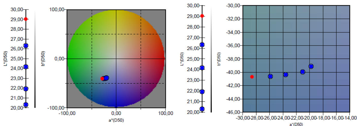
Slika 172 CIELAB prikaz transmisijskih svojstava ispitnih uzoraka s cijan bojilom 2,0 mm – 2,8 mm
