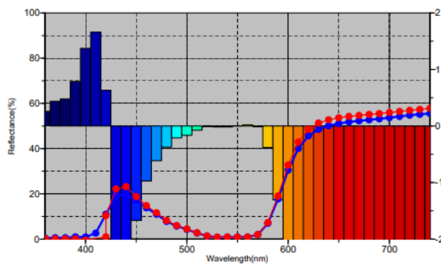
Slika 37 Spektralna krivulja transmisijskog svojstva ispitnog uzorka
