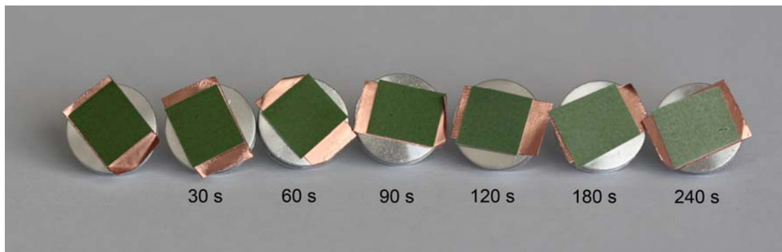
Slika 27. Nejetkan i jetkani SicpaGreen-33 uzorci pripremljeni za SEM sa označenim vremenom jetkanja (prvi uzorak na slici nije jetkan)
